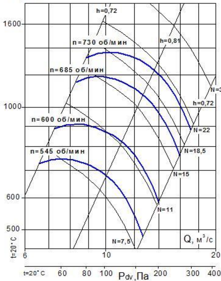
P_v , Па ВР 80-70-12,5 (исп. 1 и 5)
