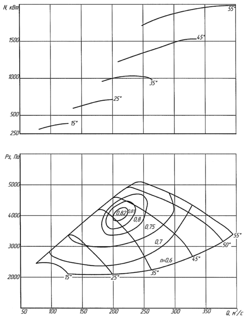
Аэродинамическая характеристика вентилятора ВО-30К. Схема М-23. Частота вращения 750 об/мин.
