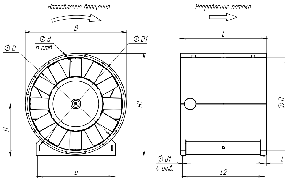
Тип крепления - 02 (на опоре)
