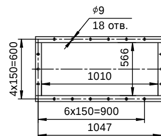
Выходной фланец
