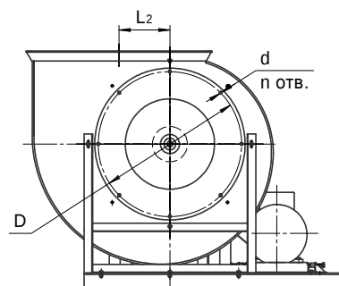
Выходной фланец
