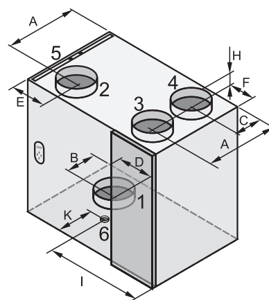
Подсоединения 3/1 R
