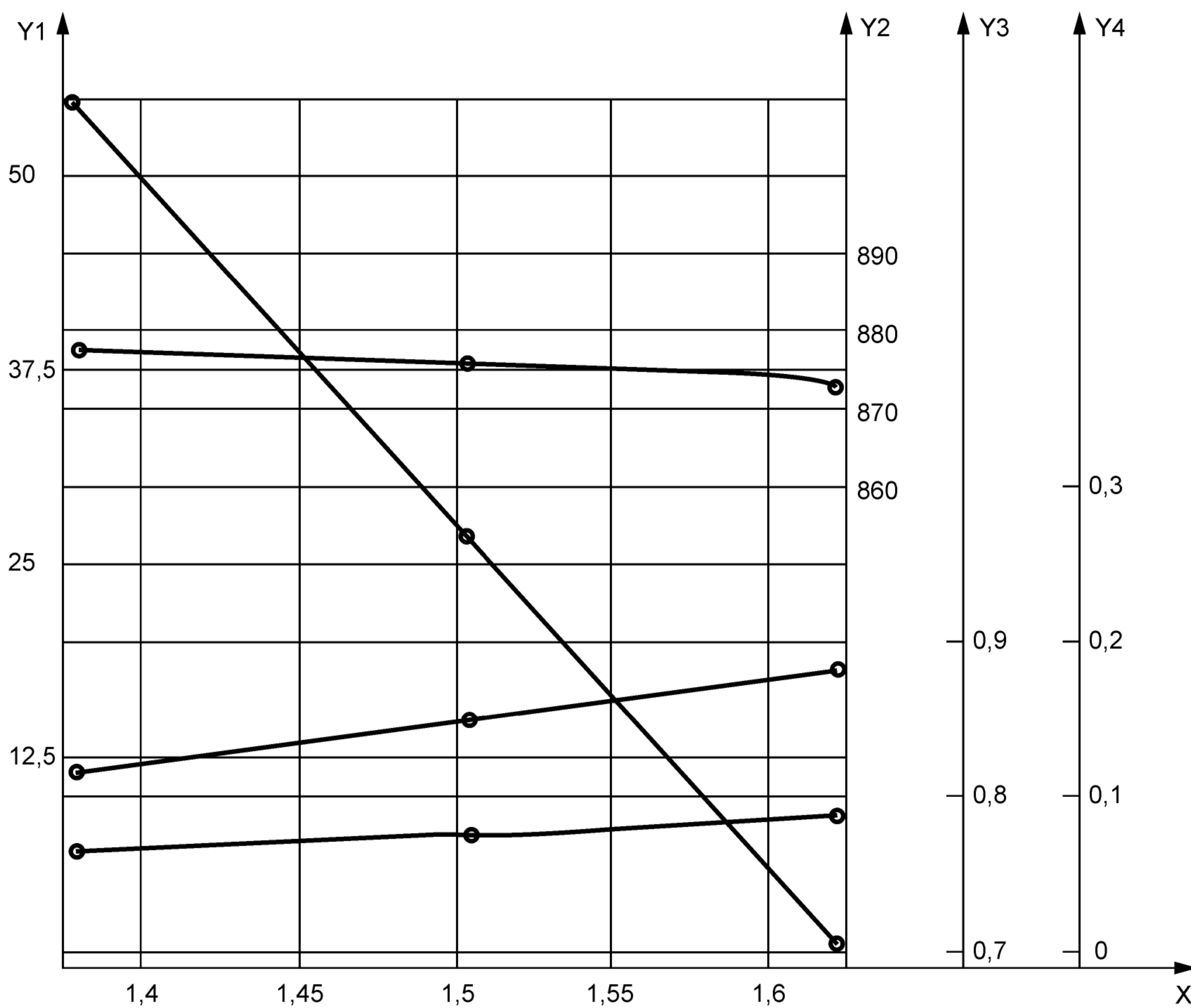
X — расход воздуха АСУ (м³/с); Y1 — статическое давление (Па); Y2 — скорость вентилятора (об/мин); Y3 — потребляемая мощность (кВт); Y4 — эффективность на единицу
